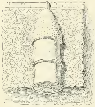
49. — Partie supérieure du drainage d'un tertre, vue perspective.
